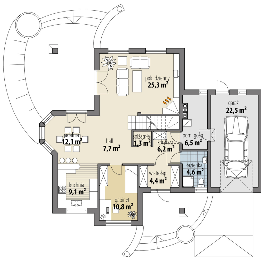
RZUT PARTER
