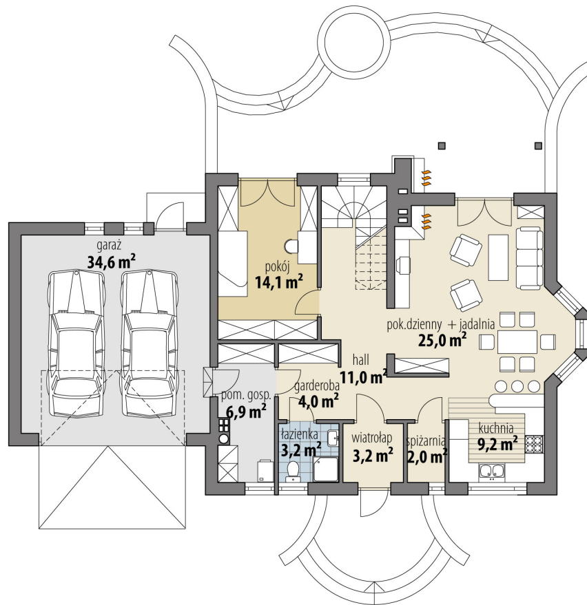
RZUT PARTER
