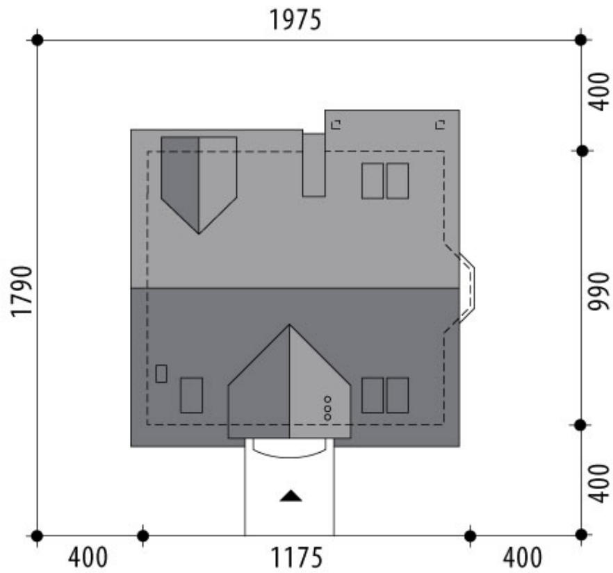
RZUT DZIAŁKI
