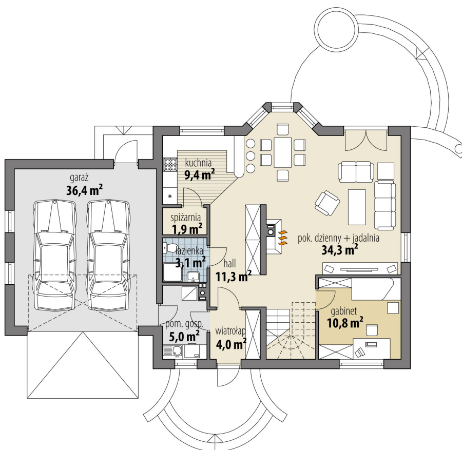
RZUT PARTER
