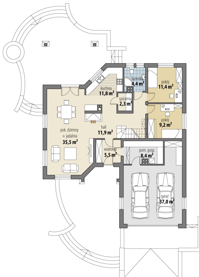
RZUT PARTER
