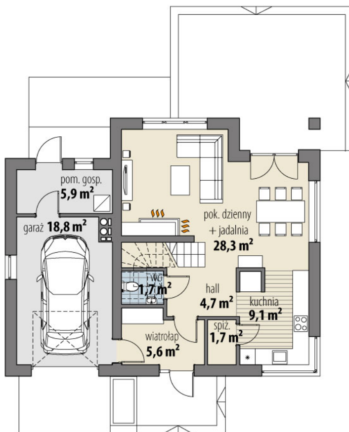
RZUT PARTER
