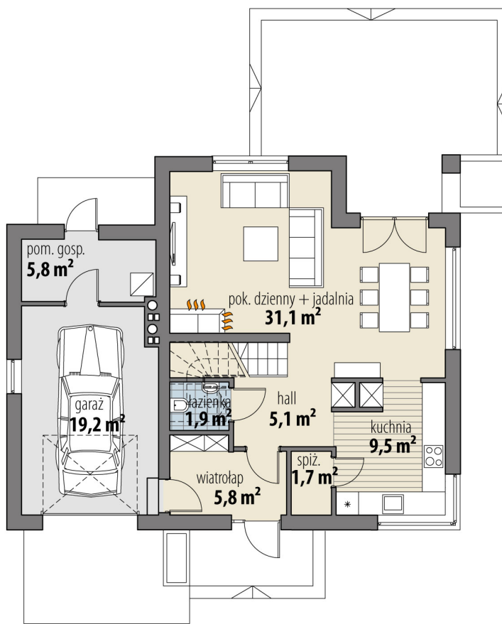
RZUT PARTER
