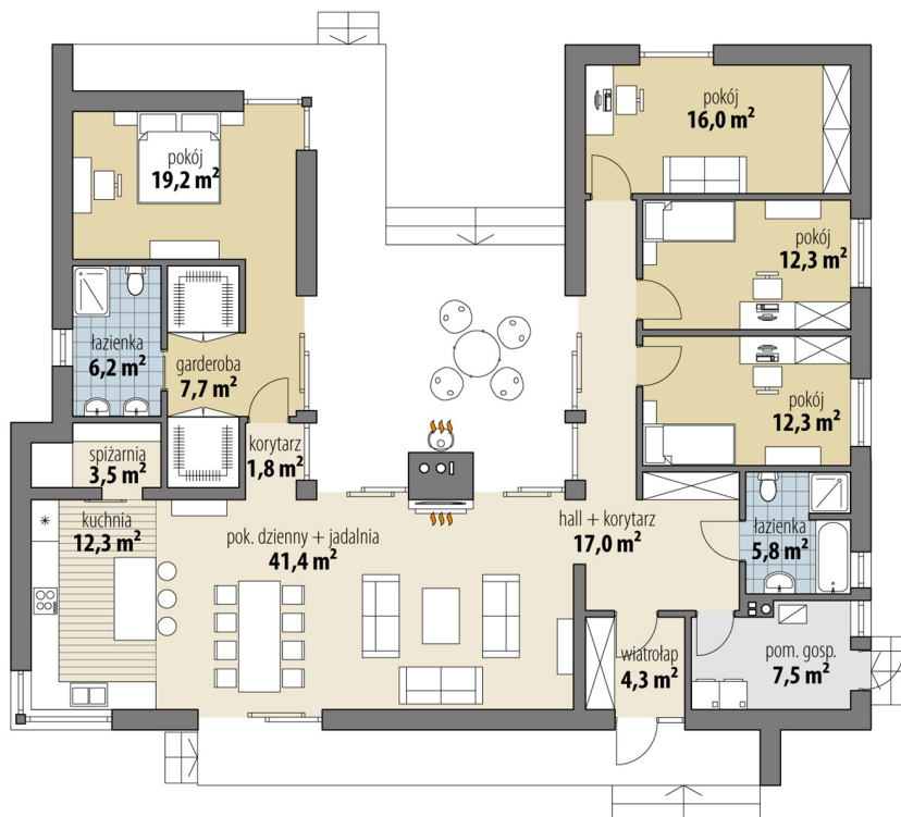
RZUT PARTER
