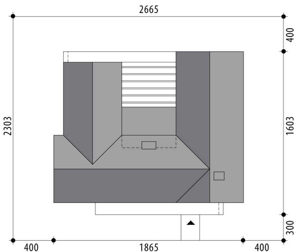
RZUT DZIAŁKI
