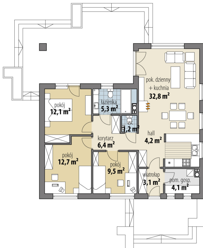
RZUT PARTER
