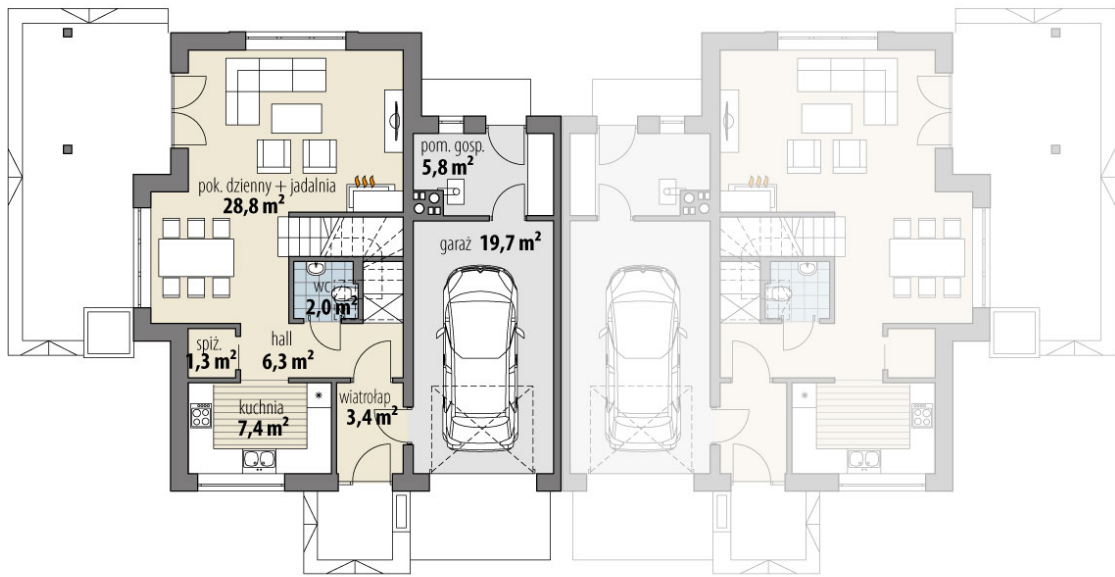
RZUT PARTER
