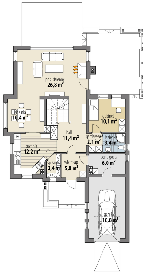
RZUT PARTER
