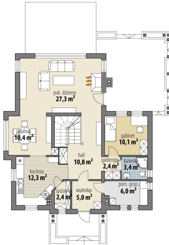
RZUT PARTER
