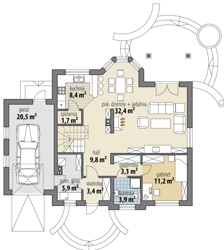
RZUT PARTER
