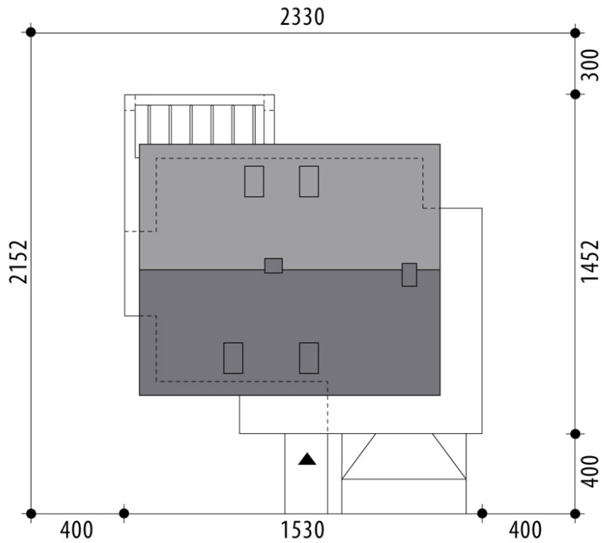
RZUT DZIAŁKI
