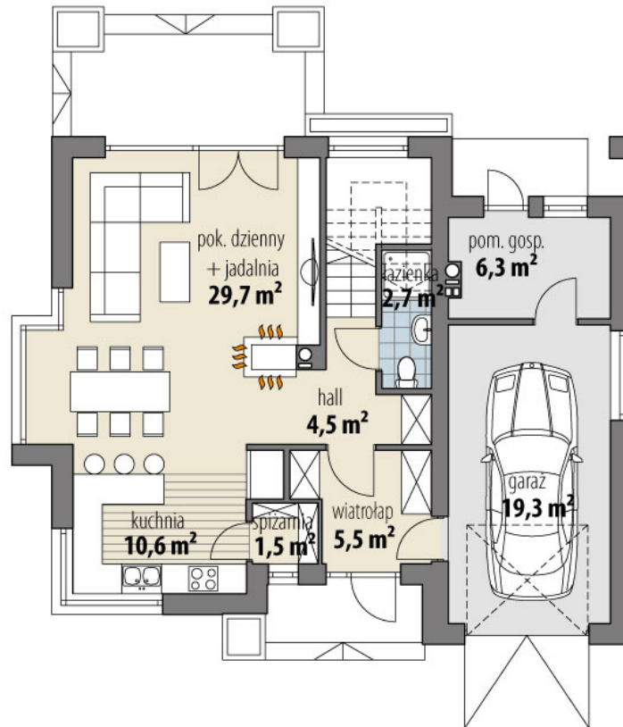
RZUT PARTER
