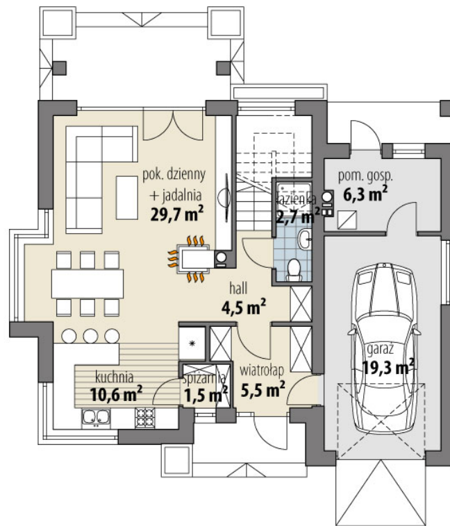
RZUT PARTER
