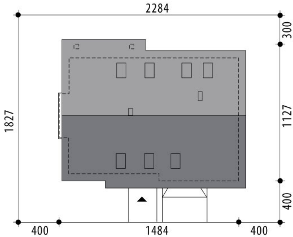
RZUT DZIAŁKI
