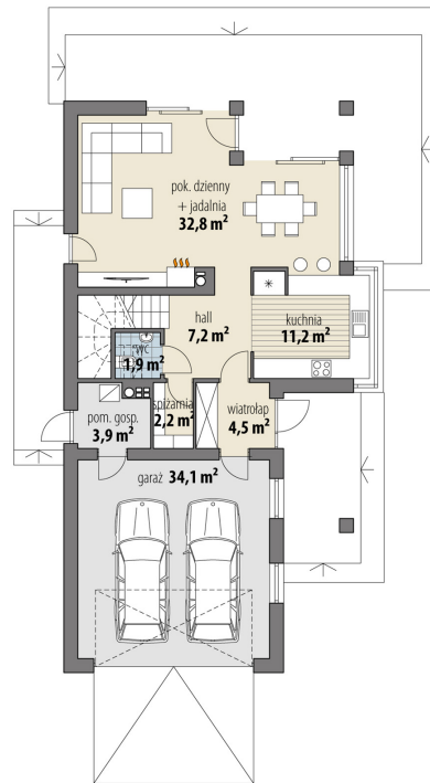
RZUT PARTER
