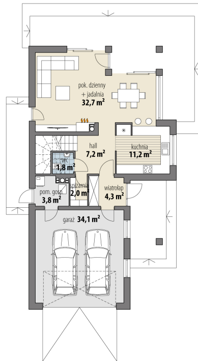
RZUT PARTER
