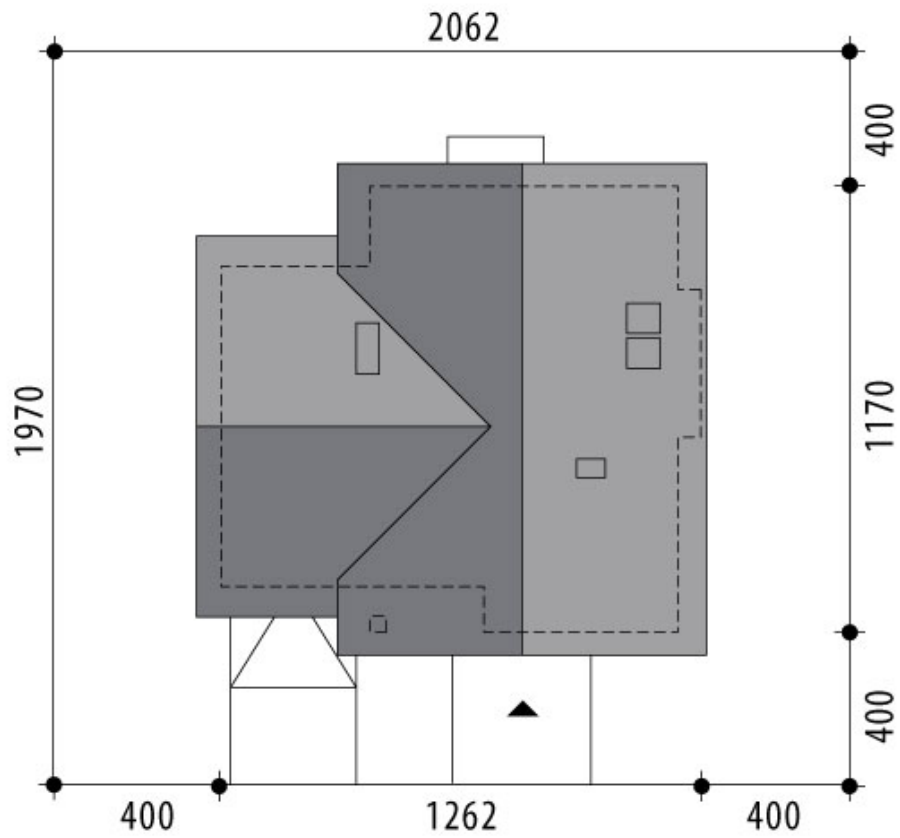
RZUT DZIAŁKI
