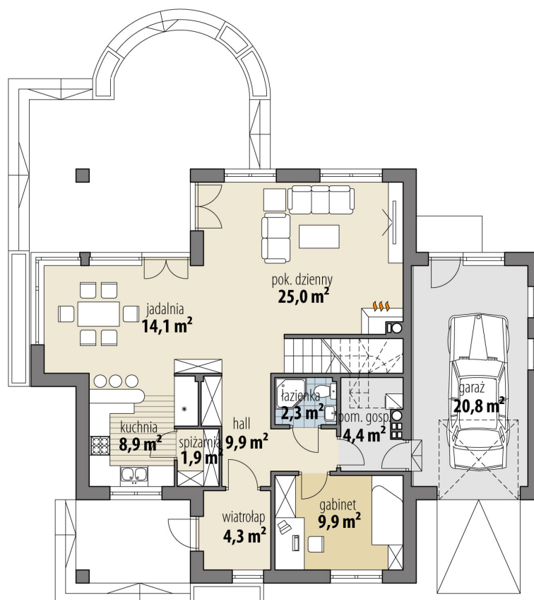
RZUT PARTER
