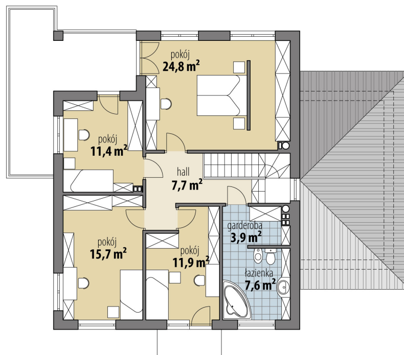
RZUT
