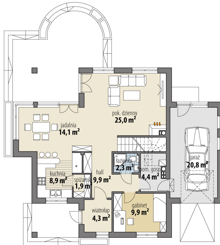
RZUT PARTER
