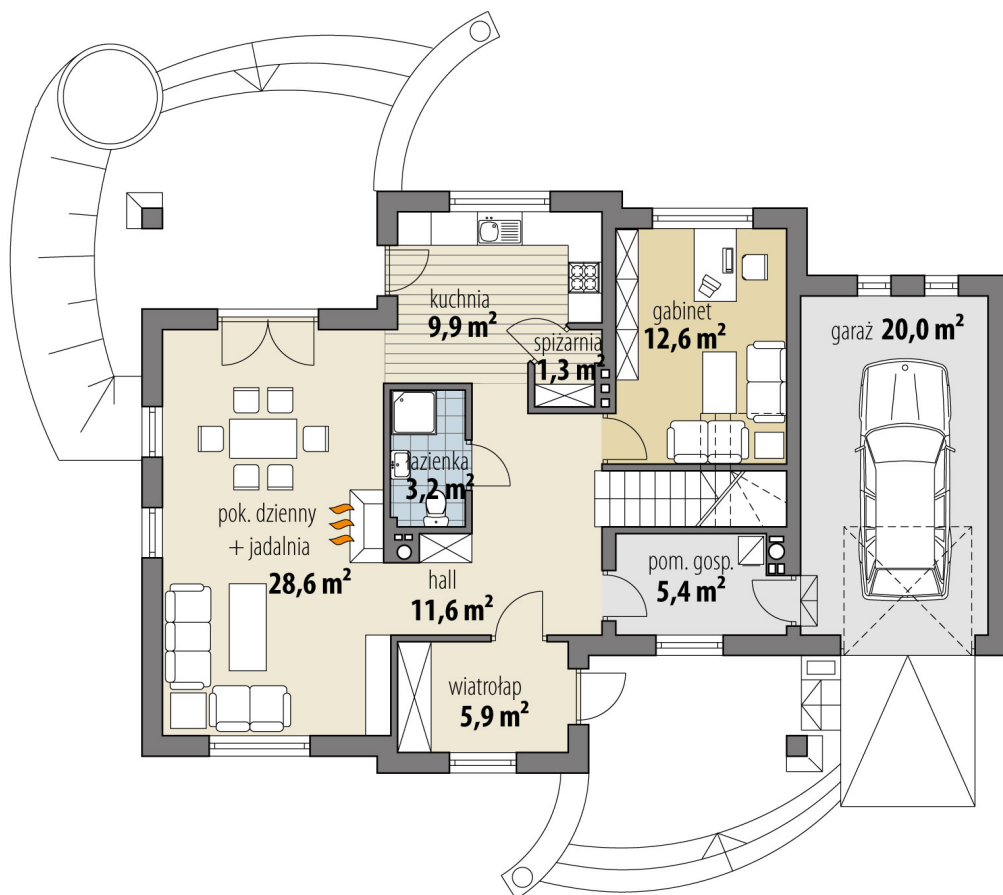
RZUT PARTER
