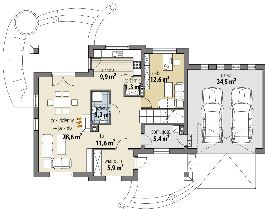
RZUT PARTER
