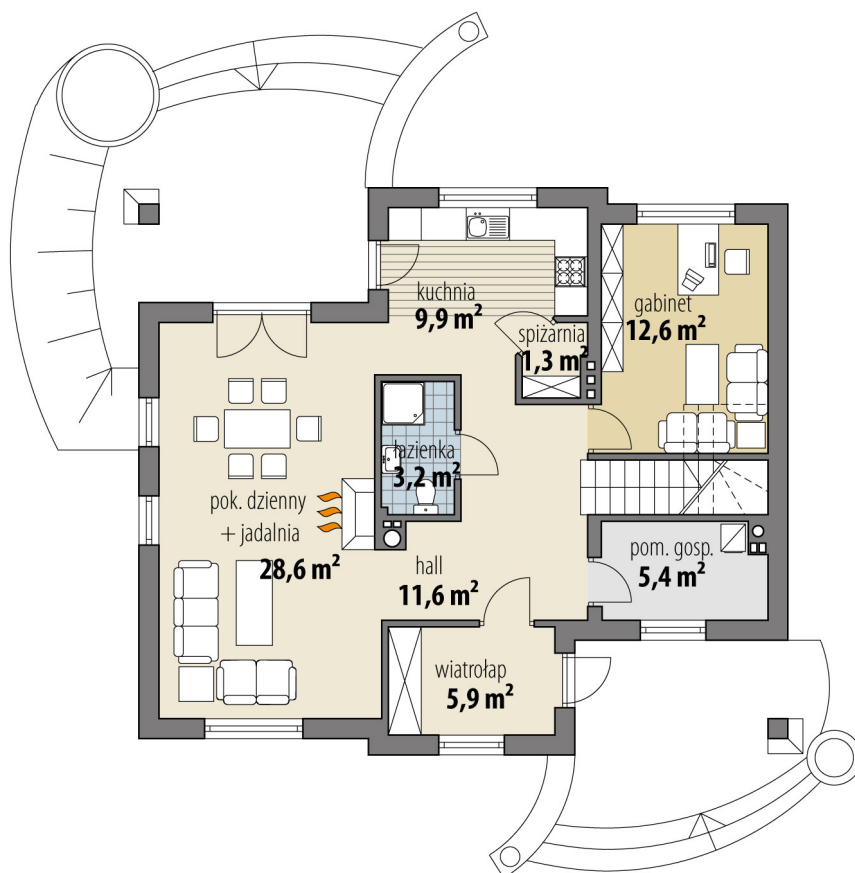
RZUT PARTER
