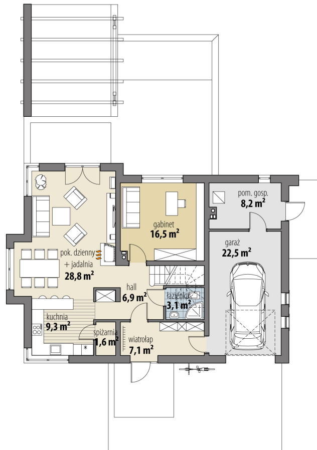
RZUT PARTER
