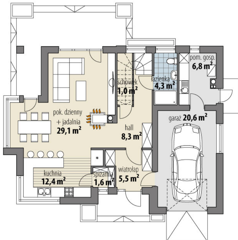
RZUT PARTER
