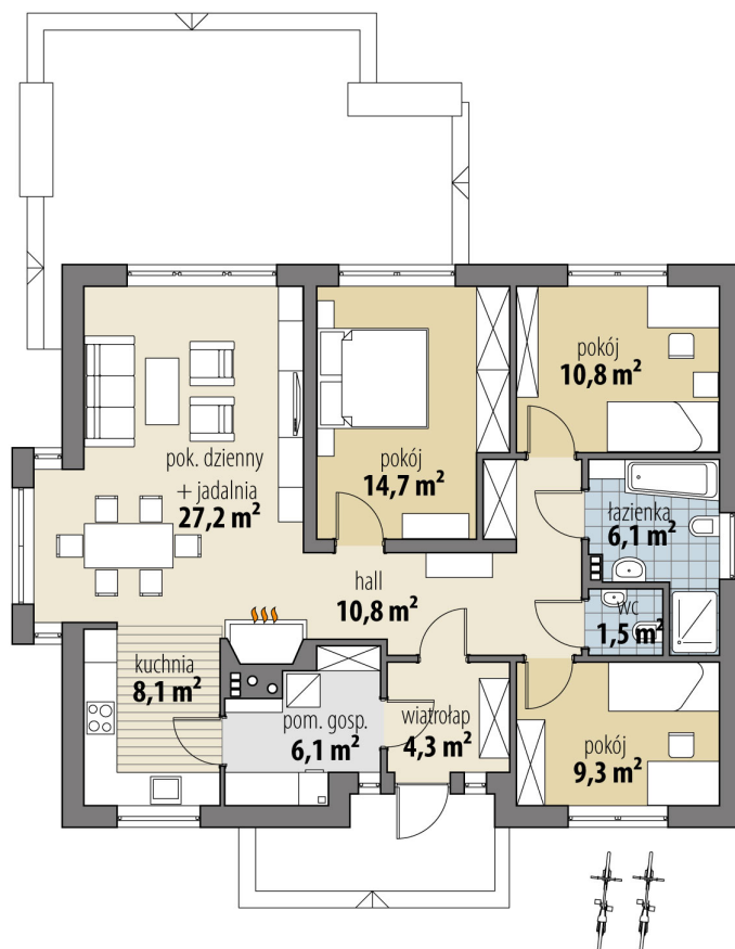
RZUT PARTER
