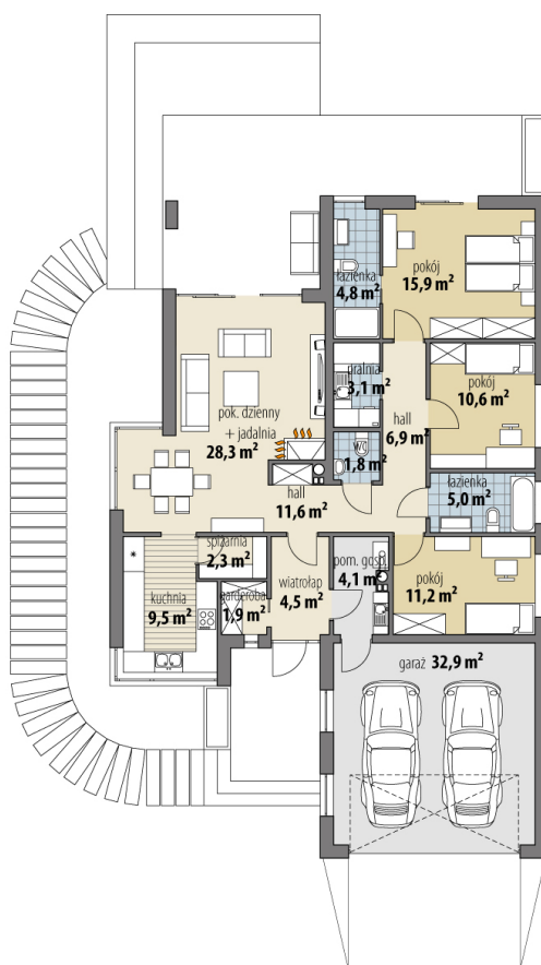
RZUT PARTER
