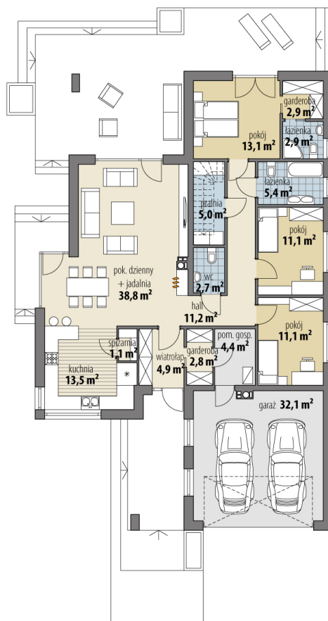
RZUT PARTER
