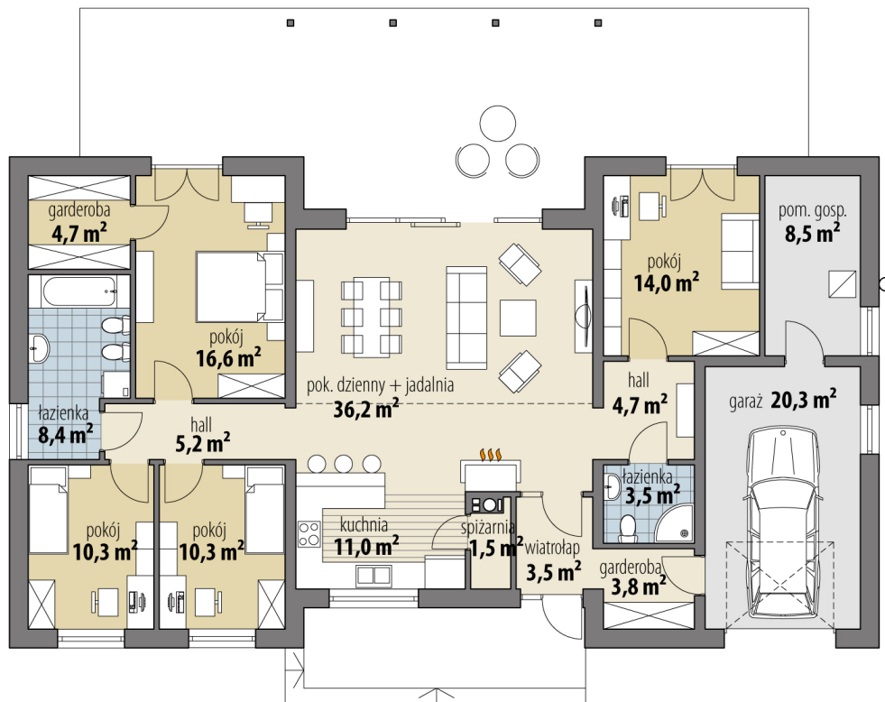
RZUT PARTER
