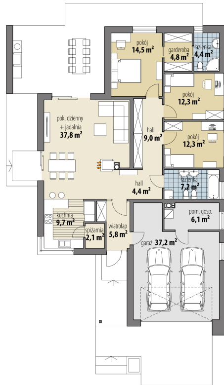
RZUT PARTER
