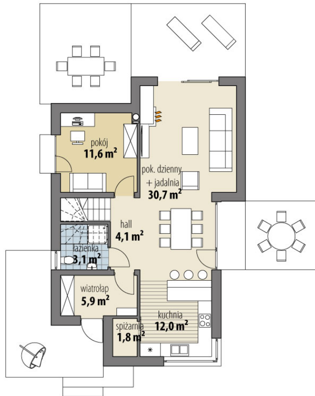
RZUT PARTER
