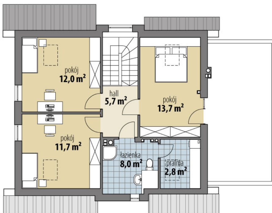
RZUT
