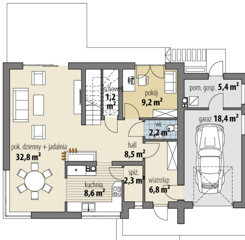
RZUT PARTER
