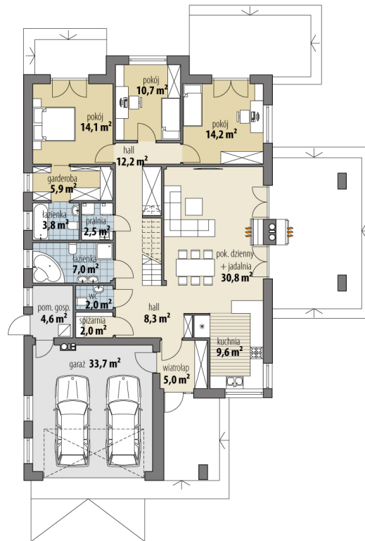
RZUT PARTER
