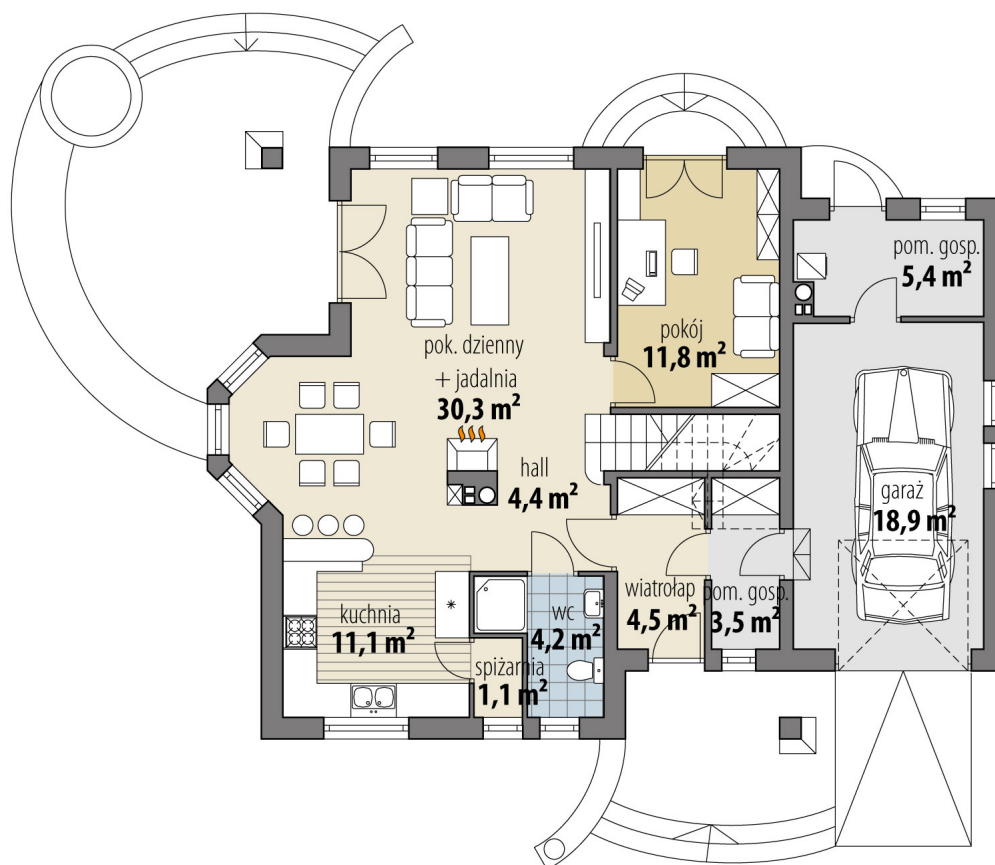
RZUT PARTER
