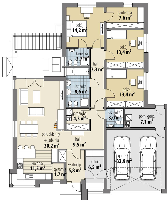
RZUT PARTER
