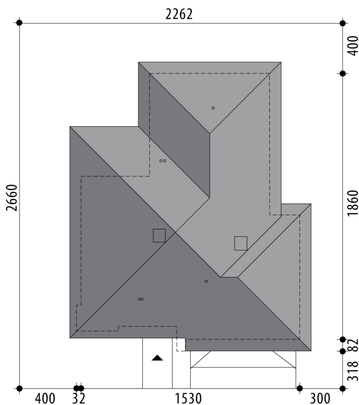
RZUT DZIAŁKI
