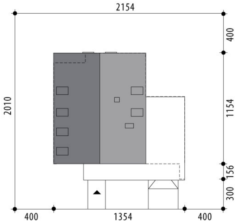
RZUT DZIAŁKI
