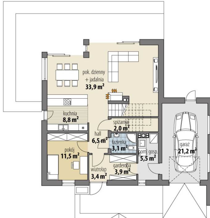
RZUT PARTER
