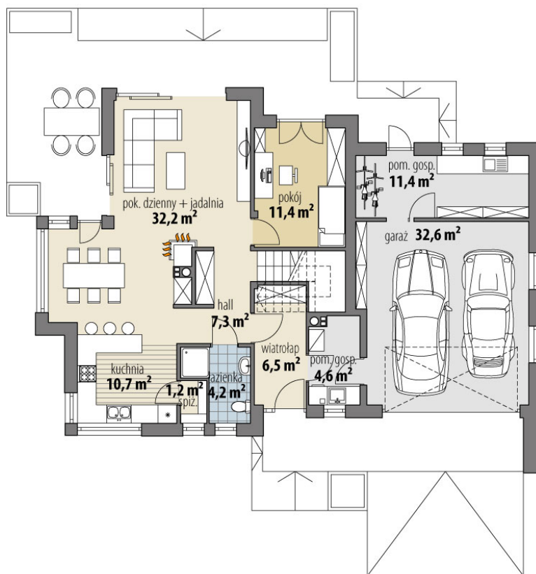
RZUT PARTER
