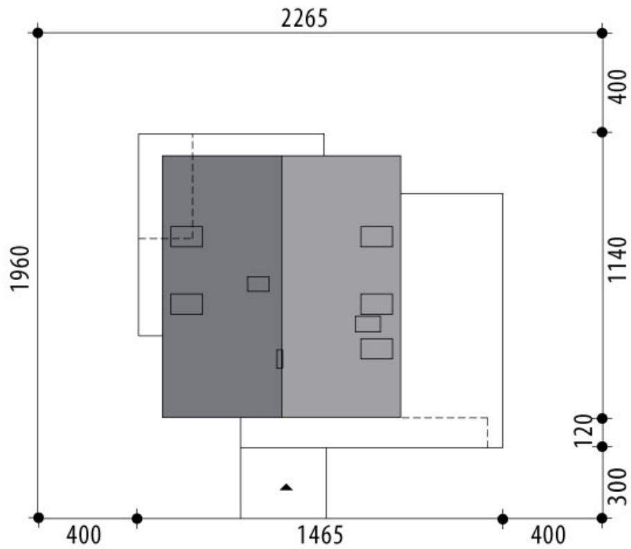
RZUT DZIAŁKI
