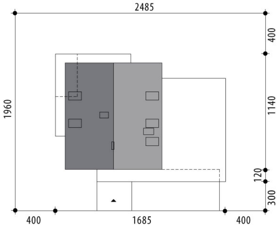
RZUT DZIAŁKI
