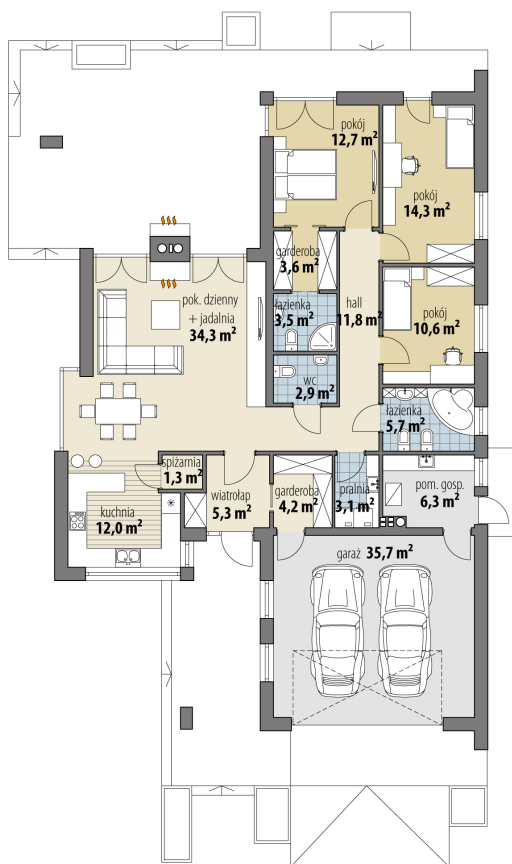
RZUT PARTER
