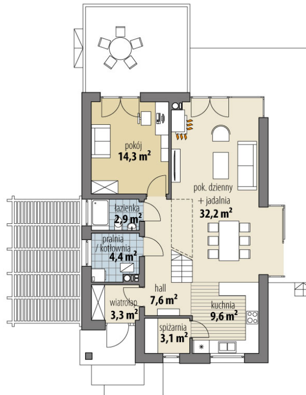
RZUT PARTER
