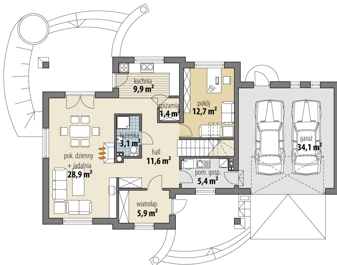
RZUT PARTER
