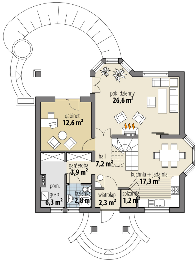
RZUT PARTER
