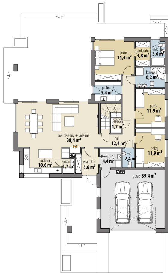
RZUT PARTER
