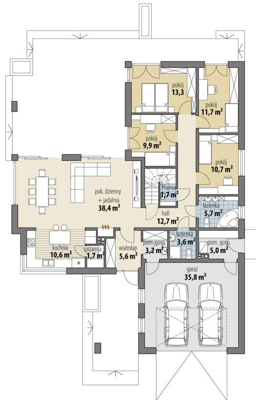
RZUT PARTER
