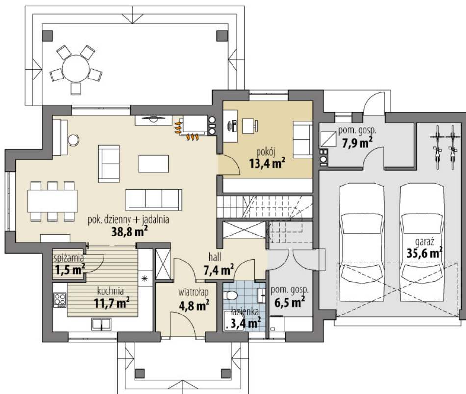
RZUT PARTER
