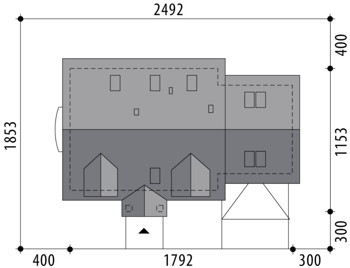
RZUT DZIAŁKI
