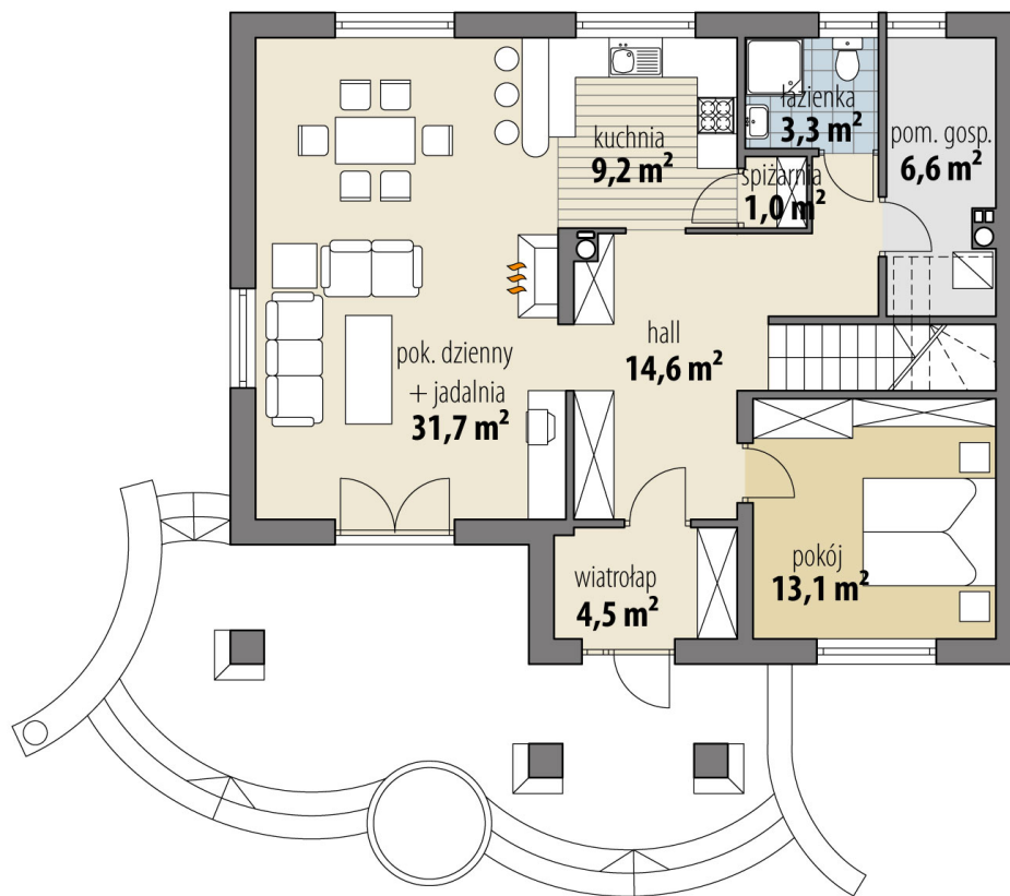
RZUT PARTER
